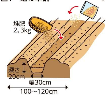
図2 3本仕立て
