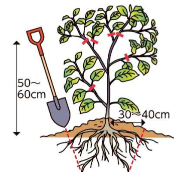
図4 更新剪定
